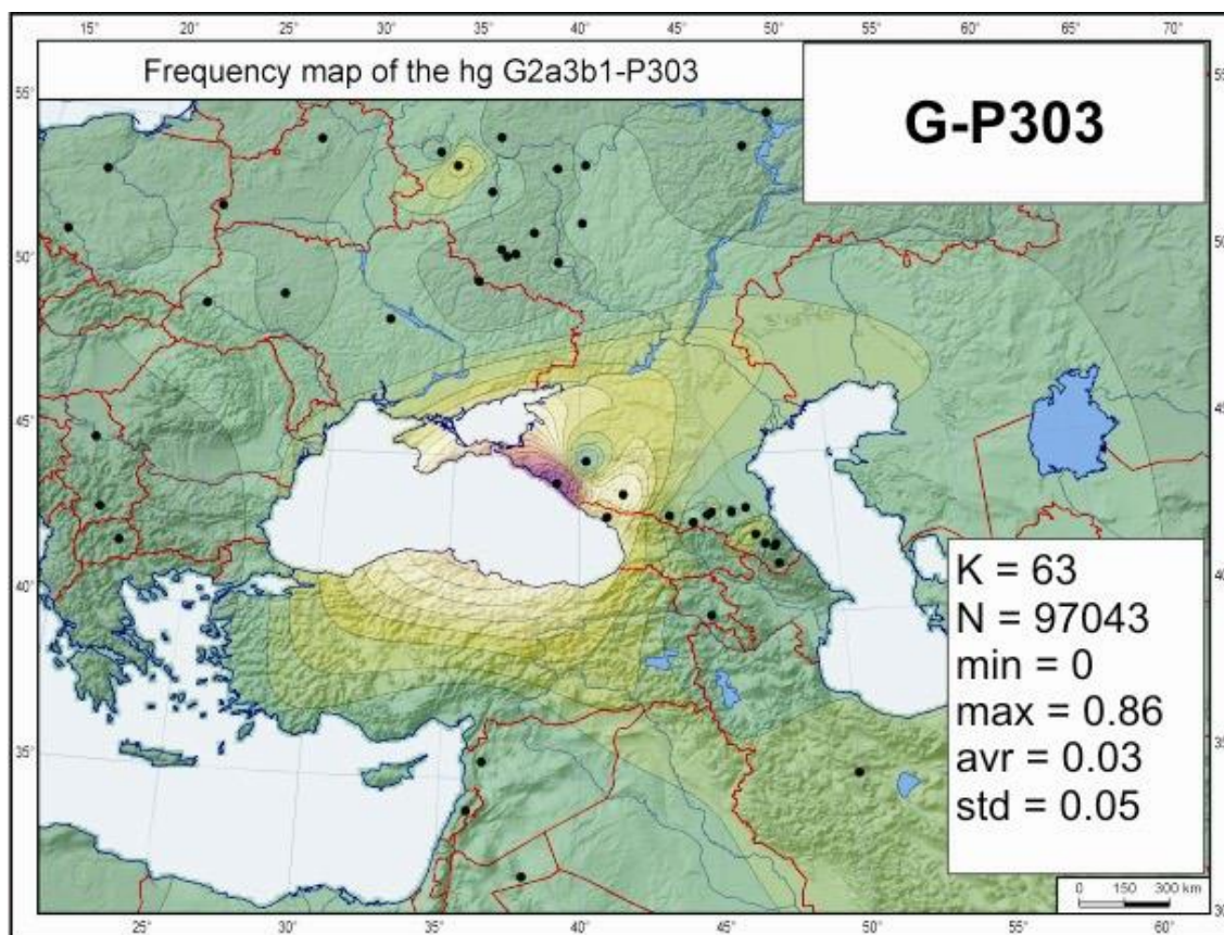
Рис.3. Частоты гаплогруппы G2a3b-P303
